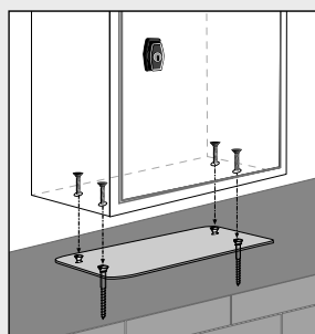
Piastra per PaccoBoxXL e Modular LP
