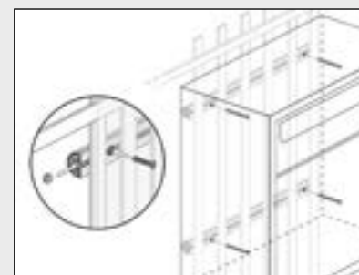
Traversini per PaccoBoxXL, EasyBox Vano Unico, ModularLP e EasyBox
