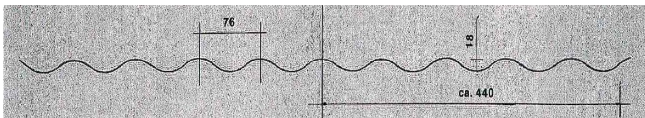
Desen 1 : Dimensiuni profilului ondulat 76 x 18 mm
