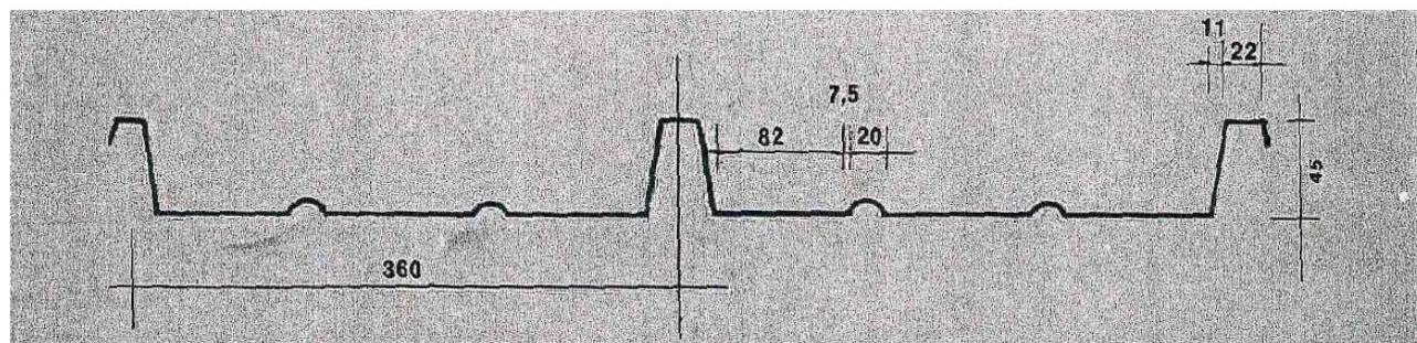
Desen 2 : Dimensiuni profilului cutat cu 3 grinzi
