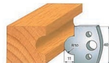
Cod cutit Art. SA0014 - (SA1014) cod contracutit
