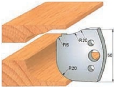
Cod cutit Art. SA2061 - (SA3061) cod contracutit
