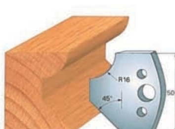
Cod cutit Art. SA2053 - (SA3053)cod contracutit
