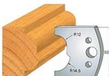
Cod cutit Art. SA2020 - (SA3020)cod contracutit
