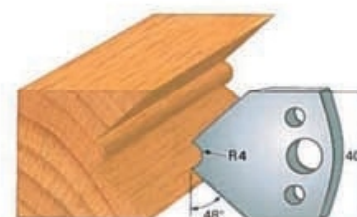
Cod cutit Art. SA0080 - (SA1080)cod contracutit
