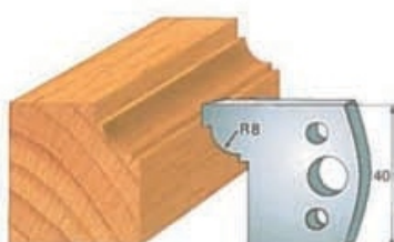
Cod cutit Art. SA0067 - (SA1067)cod contracutit
