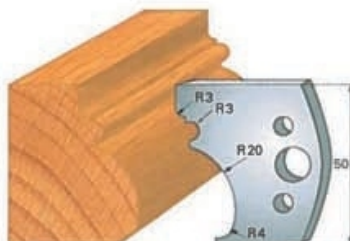
Cod cutit Art. SA2001 - (SA3001)cod contracutit
