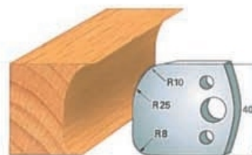
Cod cutit Art. SA0062 - (SA1062)cod contracutit
