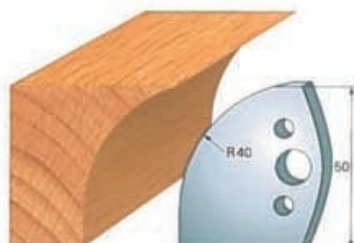
Cod cutit Art. SA2049 - (SA3049)cod contracutit
