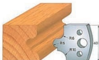
Cod cutit Art. SA0012 - (SA1012) cod contracutit
