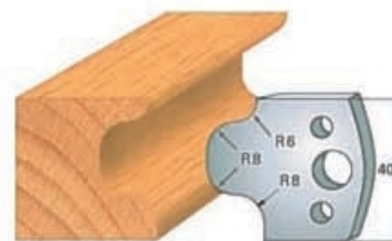
Cod cutit Art. SA0056 - (SA1056)cod contracutit
