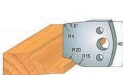
Cod cutit Art. SA0100 - (SA1100) cod contracutit
