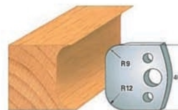
Cod cutit Art. SA0050 - (SA1050)cod contracutit
