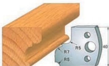
Cod cutit Art. SA0082 - (SA1082)cod contracutit
