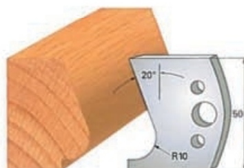
Cod cutit Art. SA2059 - (SA3059)cod contracutit
