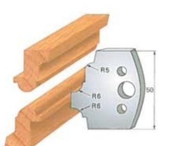
Cod cutit Art. SA2026 - (SA3026)cod contracutit
