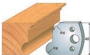
Cod cutit Art. SA0054 - (SA1054)cod contracutit
