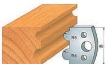
Cod cutit Art. SA0030 - (SA1030)cod contracutit
