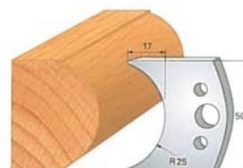
Cod cutit Art. SA2030 - (SA3030)cod contracutit
