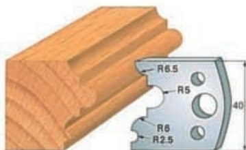
Cod cutit Art. SA0036 - (SA1036)cod contracutit
