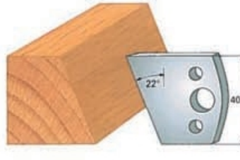
Cod cutit Art. SA0001 - (SA1001) cod contracutit
