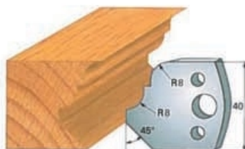
Cod cutit Art. SA0073 - (SA1073)cod contracutit
