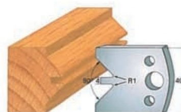
Cod cutit Art. SA0071 - (SA1071)cod contracutit
