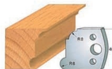
Cod cutit Art. SA0053 - (SA1053)cod contracutit
