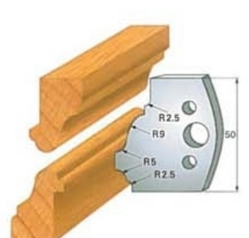
Cod cutit Art. SA2042 - (SA3042)cod contracutit
