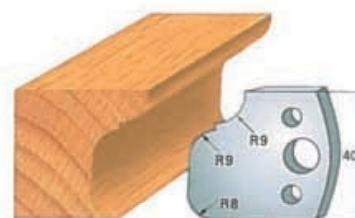
Cod cutit Art. SA0068 - (SA1068)cod contracutit
