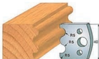
Cod cutit Art. SA0006 - (SA1006) cod contracutit
