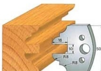
Cod cutit Art. SA2023 - (SA3023)cod contracutit
