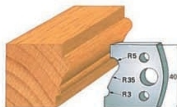
Cod cutit Art. SA0081 - (SA1081)cod contracutit
