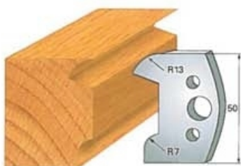
Cod cutit Art. SA2019 - (SA3019)cod contracutit
