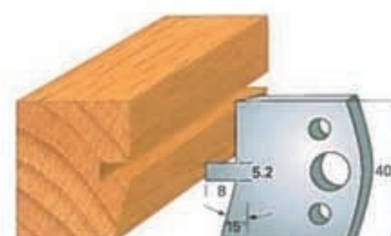
Cod cutit Art. SA0086 - (SA1086)cod contracutit
