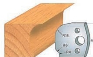
Cod cutit Art. SA0047 - (SA1047)cod contracutit
