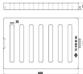
SEL ANKO-GG-207 Grătar apă pluvială 460 mm x 660 mm
