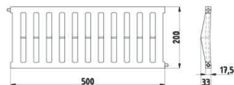
SEL ANKO-GG-208 Grătar apă pluvială 200 mm x 500 mm
