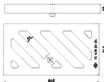
SEL ANKO-GG-201 Grătar apă pluvială 640 mm x 345 mm
