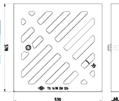
SEL ANKO-GG-200 Grătar apă pluvială 570 mm x 570 mm
