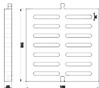
SEL ANKO-GG-204 Grătar apă pluvială 600 mm x 600 mm
