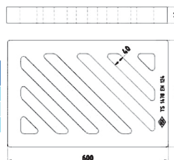
SEL ANKO-GG-203 Grătar apă pluvială 400 mm x 600 mm
