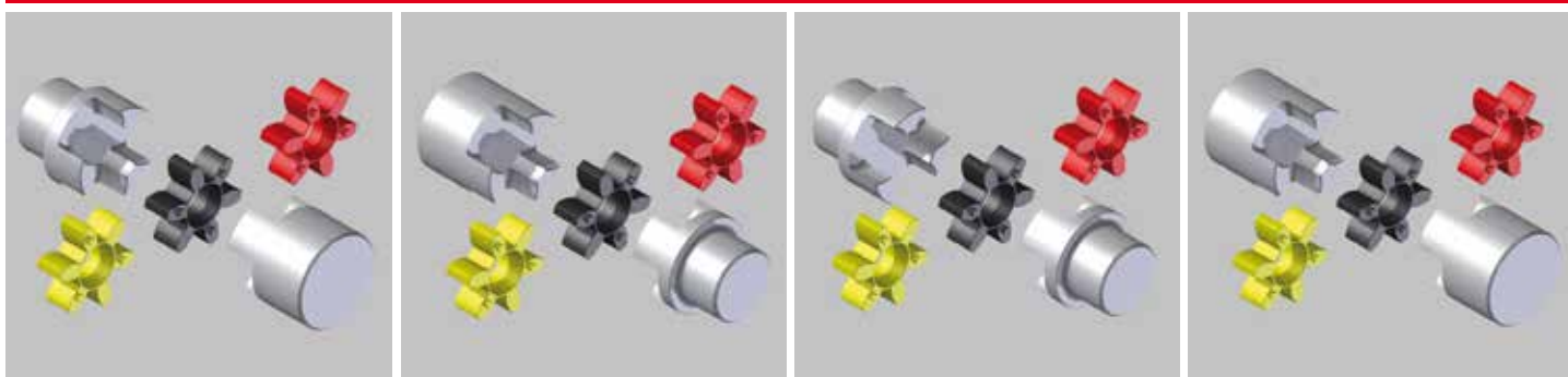
MOZZO A
