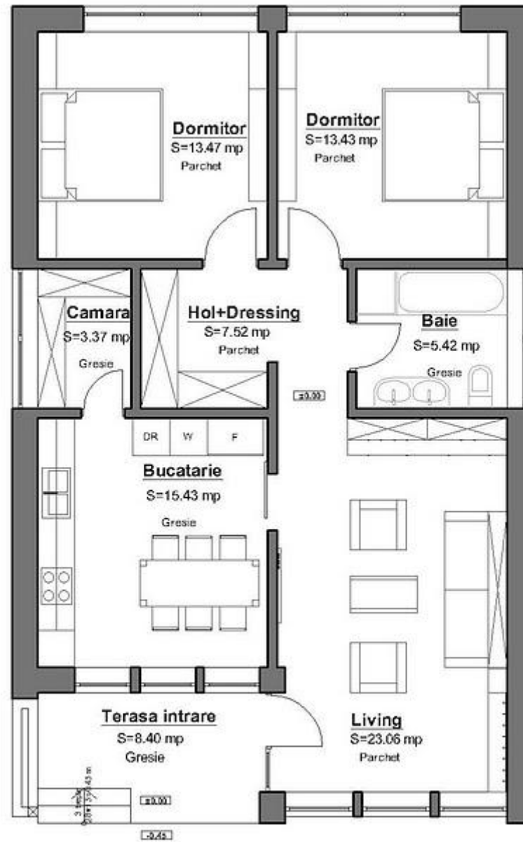
PLAN PARTER: Suprafata construita 100.00 mp Suprafata utila 81.66 mp
