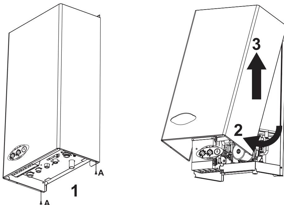
fig. 15 - Deschiderea carcasei
