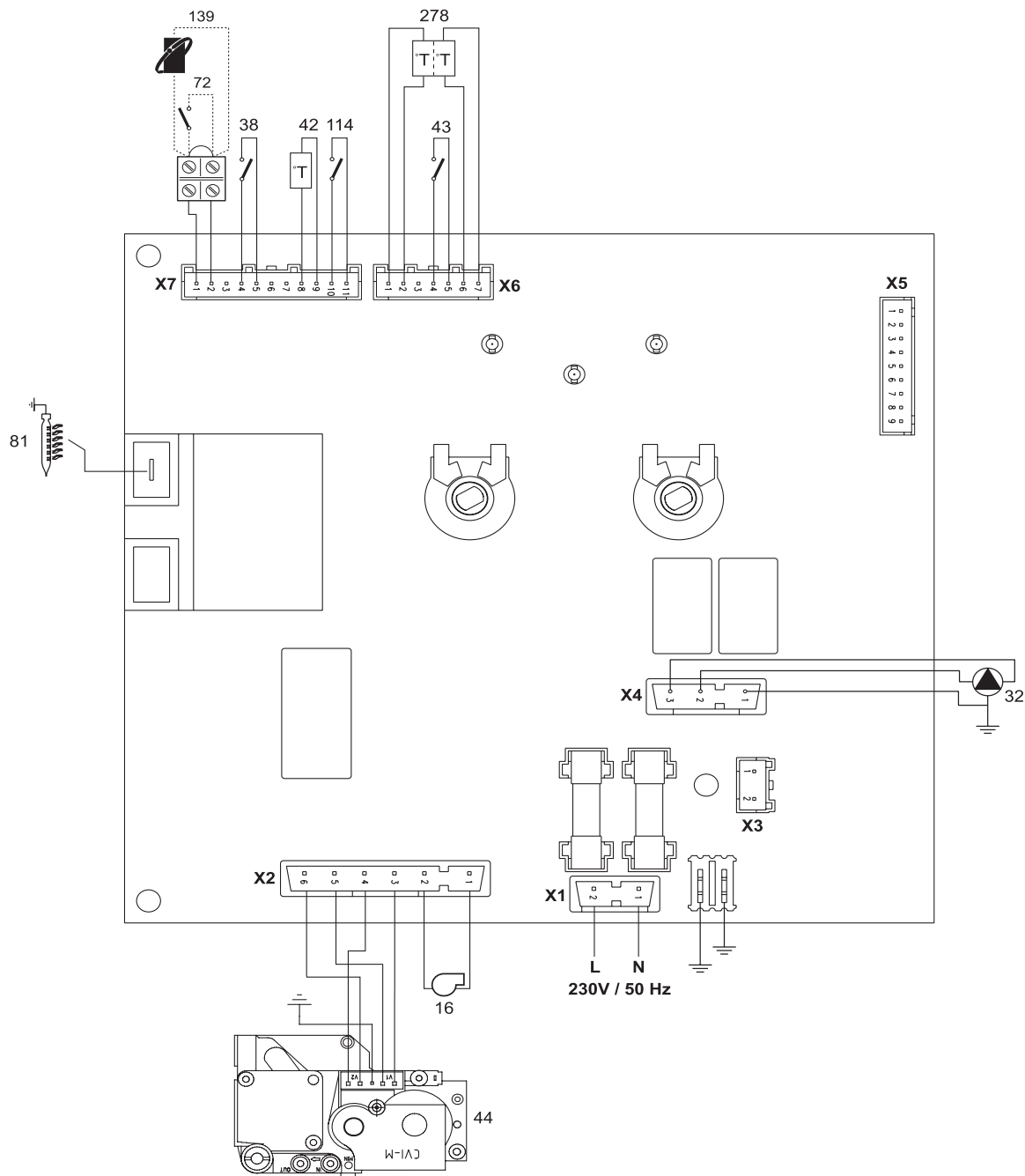
fig. 20 - Schema electrică
