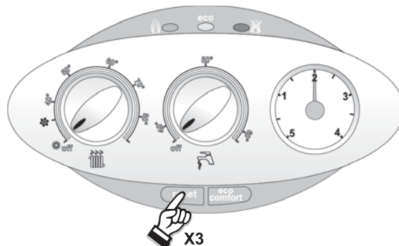
fig. 13 - Modul TEST
