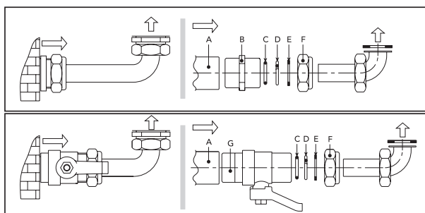
fig.5 - Kit de racordare
