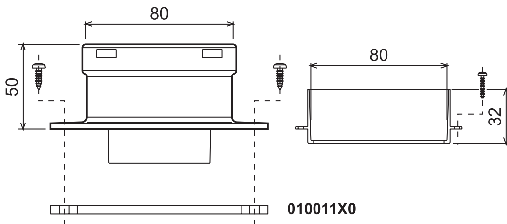
fig. 11 - Accesorii de plecare pentru conducte separate
