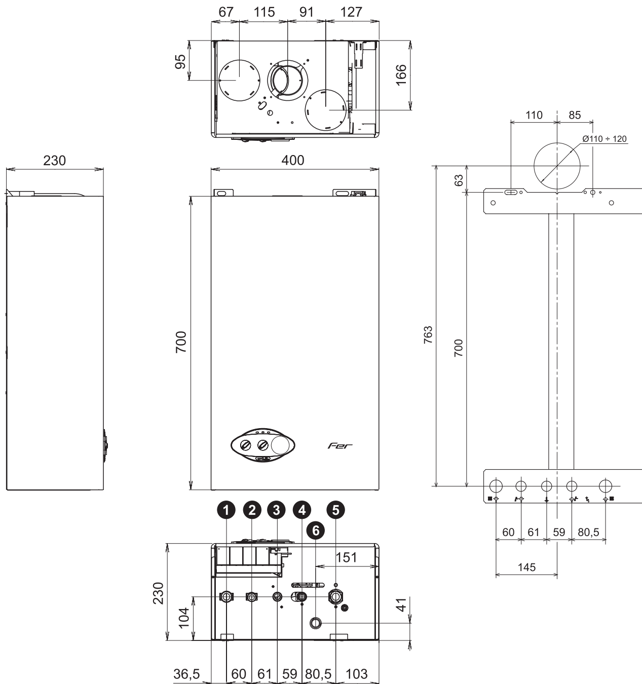
fig. 17 - Dimensiuni și racorduri
