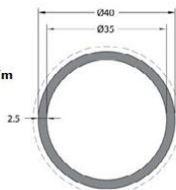
Montant \varnothing 40
