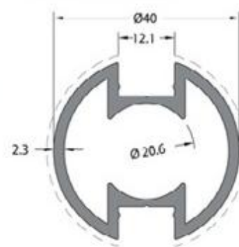
Montant \varnothing 40
