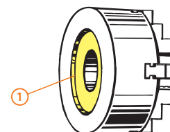
① Centrare conform DIN 6350 / 6351 (șurub de prindere din spate).
