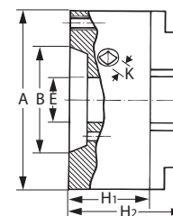
① Con scurt conform DIN 55027 (șuruburi prizoniere și piulițe cu guler).
