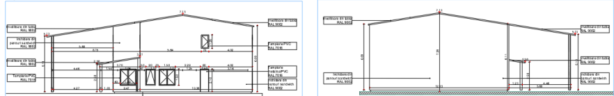
FATADA NORD SC. 1:100
