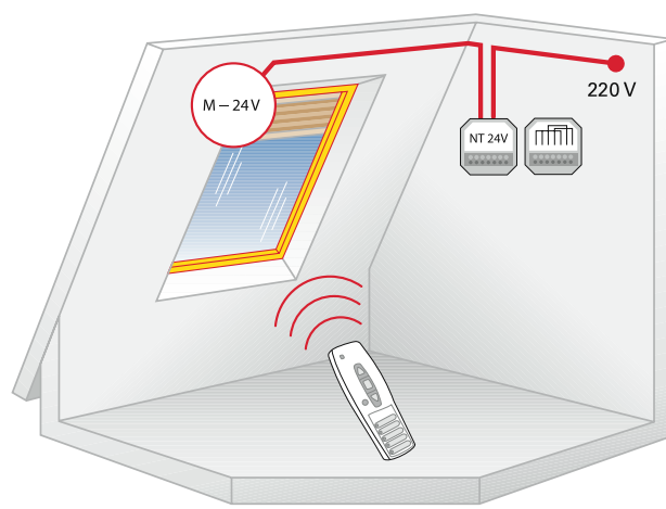
Schema de legare a motorului 24V pentru fereastra de mansardă (sau jaluza interioră sau rulouri plisante Falstore) cu acționare electrică
