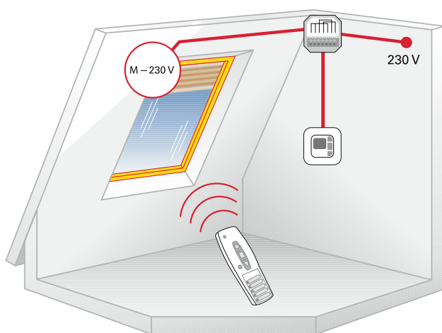
Schema de legare a motorului 230V pentru fereastra de mansardă (sau roletă exterioră sau marchiză exterioră) și întrerupător sau telecomandă
