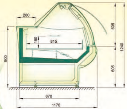
LNG-xxx-05
