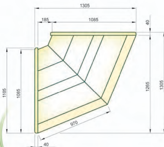
LDG-NZ90-05
