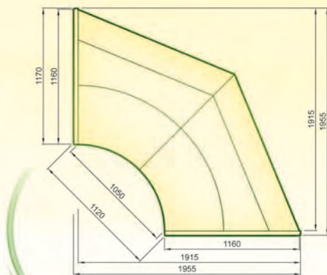
LDG-NW90-04
