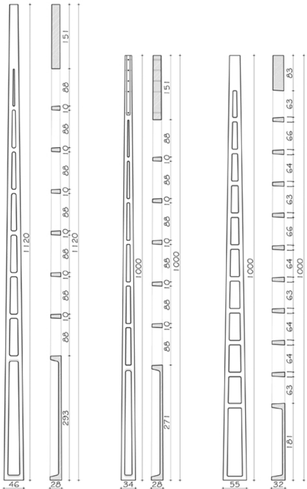
stâlp tip SE 5T
