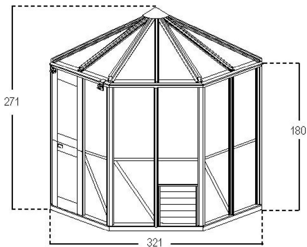
Pavilion 7,5 mp
