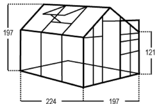
Seră hobby 4,4
