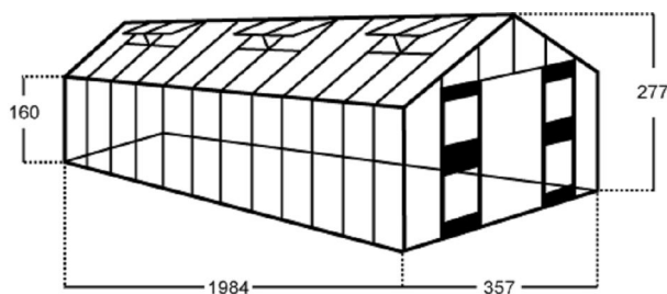
Pavilion 7,5 mp
