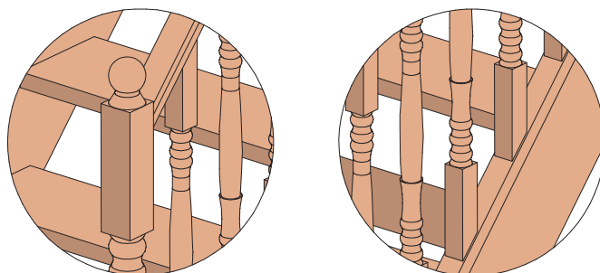
Alfa cu turnantă cu balustradă strunjită, cu contratrepte
