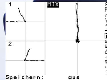
Dual Frequency Mix Mode Gleichzeitige Darstellung beider Prüfkanaäle und des Mixkanaals
