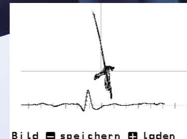
Dual Screen Rotor Mode Impedanzabbildung mit Umfangsdarstellung
