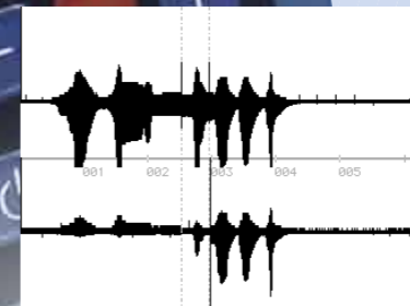
Strip Chart Mode Langzeitaufzeichnung der X- und Y-Signalkomponenten mit Rekonstruktionsmöglichkeit der Impedanzdarstellung
