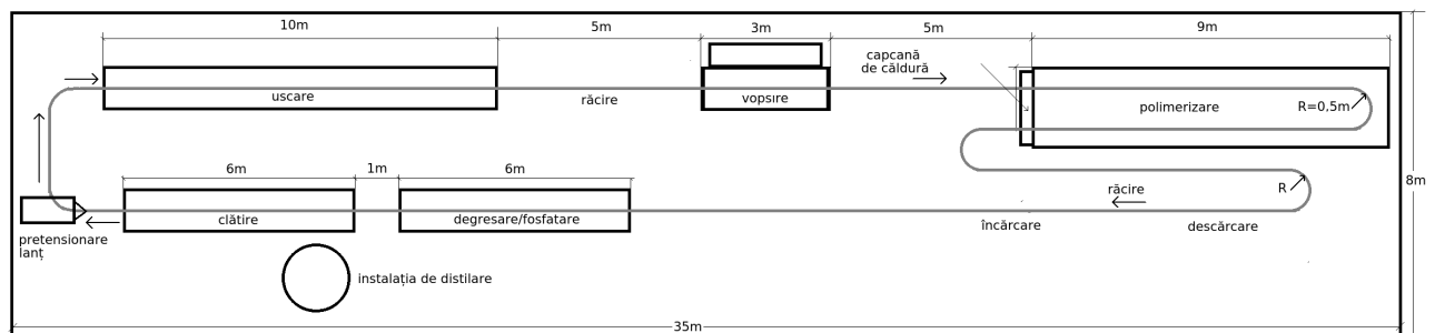
7. Confirurația liniei de conveiere automată
