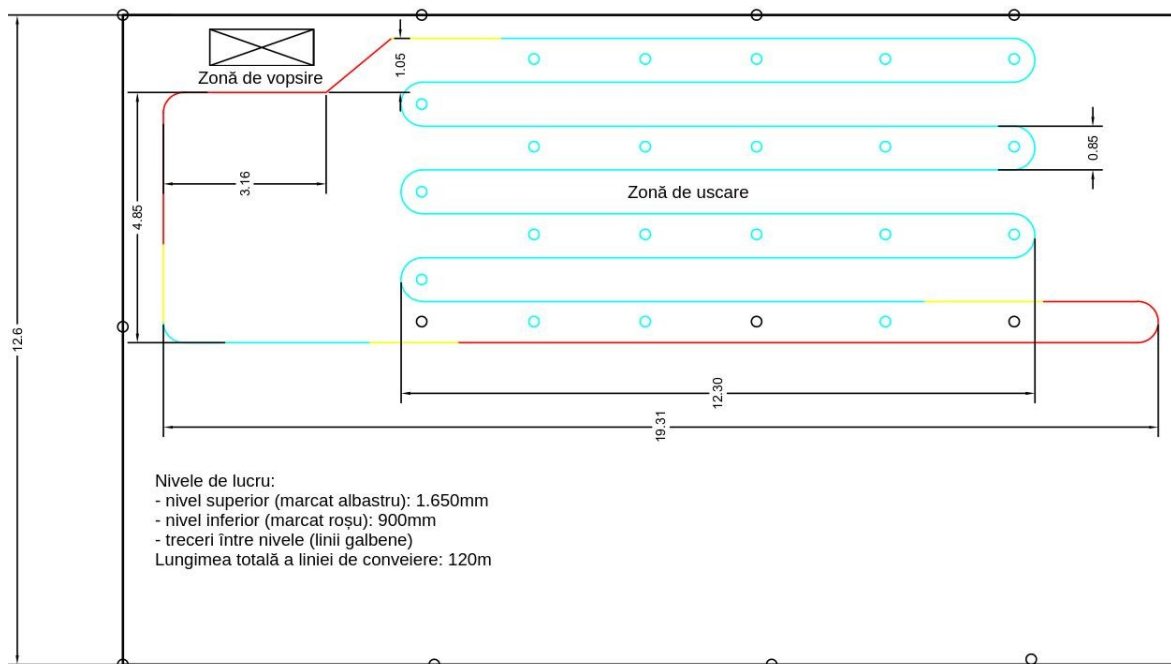
16. Configurația conveiorului automat asamblat în formă completă
