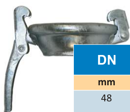
CUPLA MAMA TIP F OARBA (CAPAC) CU LEVIER SI O-RING INCLUS 1), 2)
