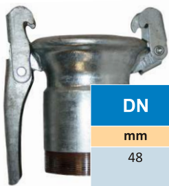
CUPLA MAMA TIP F CU LEVIER SI FILET EXTERIOR BSP 1), 2)
