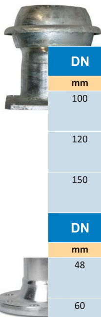
CUPLA TATA TIP F CU INEL SI FLANSA PATRATA (SAU ROTUNDA) CONFORM EN PN 10) 1), 2)
