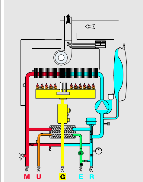
Cameră etanșă - model FF
