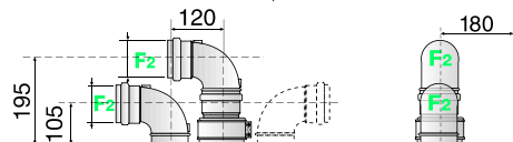
Model FF - Cameră etanșă / sistem de evacuare cu tuburi separate
