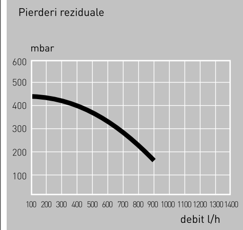
Cameră deschisă - model CF
