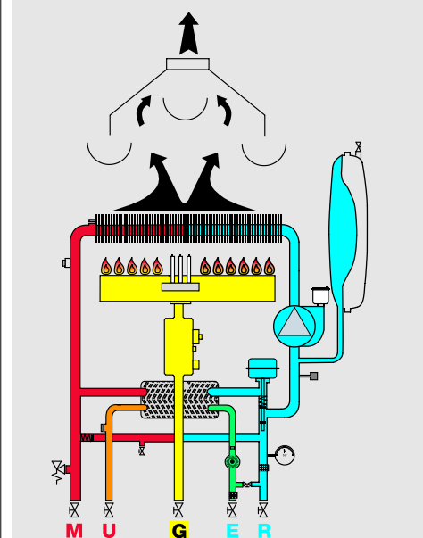
Cameră deschisă - model CF
