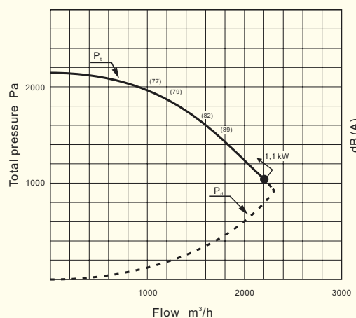
GMT 200 S, GMT 200 T
