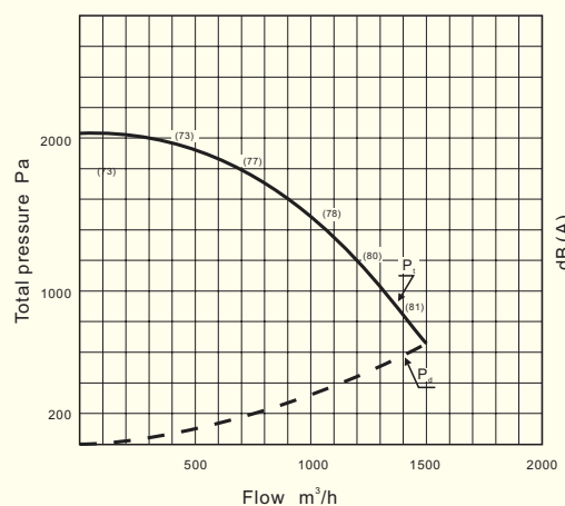
GMT 130 S, GMT 130 T
