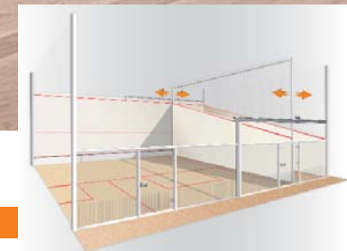
CT FLEXI Court mit verschobener Seitenwand
