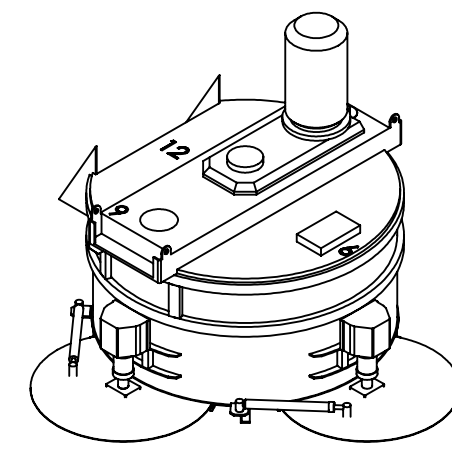
Malaxor Sicom 1125/750
