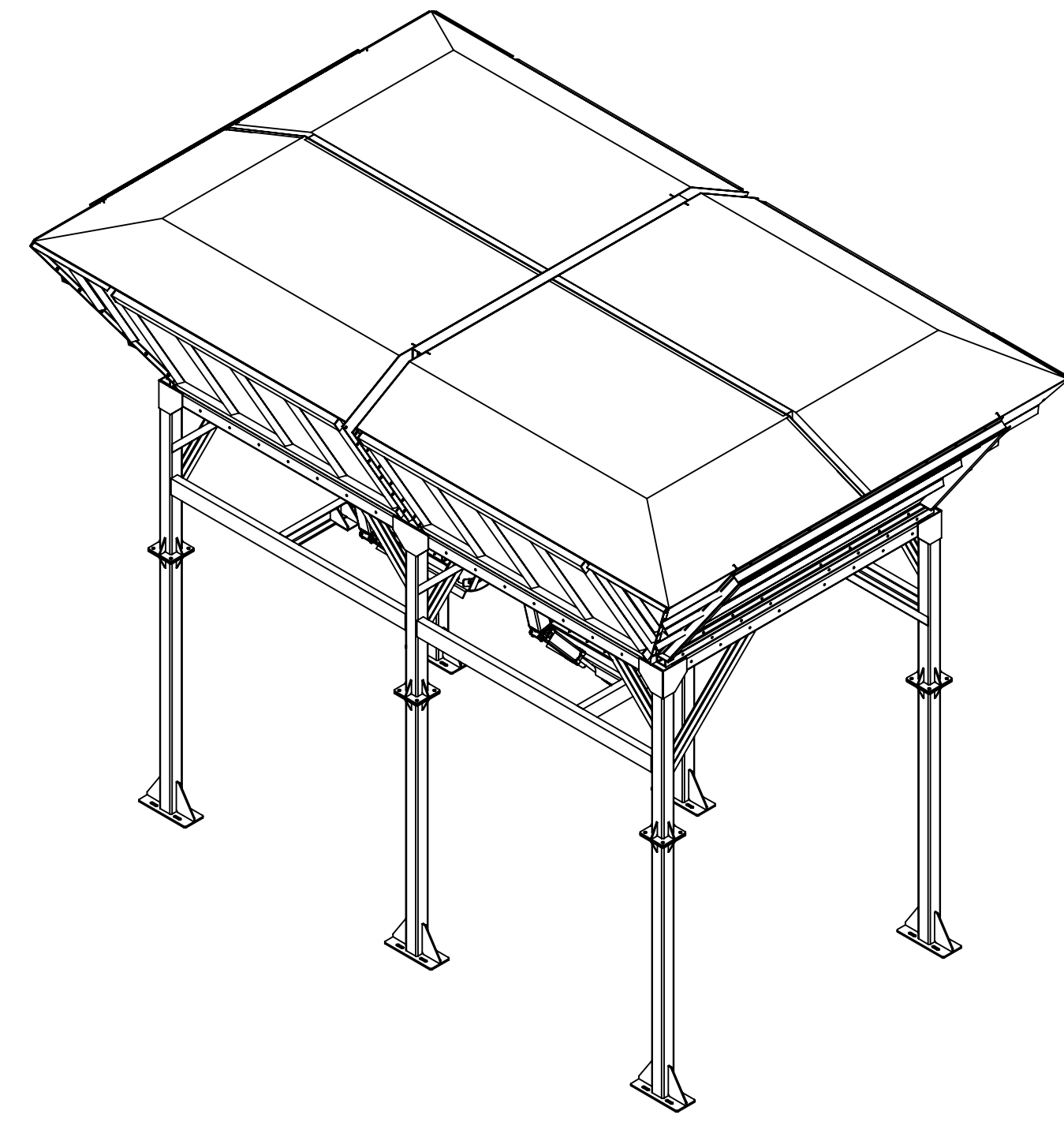
Predozare (buncar agregate)
