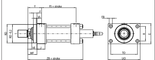
N (ISO ME5) = front flange
