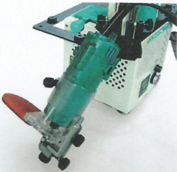
4 Fresatrice elettrica per finitura bordo Electric milling machine for edge finishing Freza de mare turatie curatire cant gros
