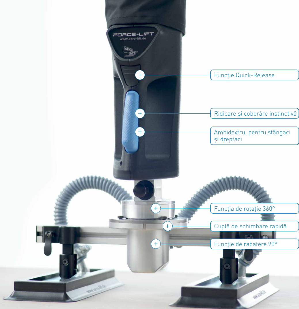
Cuplă de schimbare rapidă
