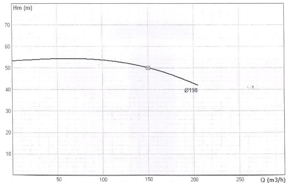
Curba de performanta
