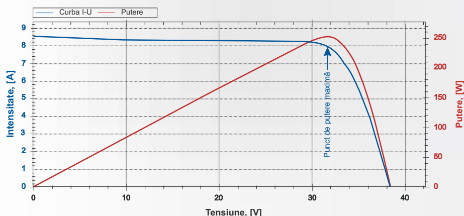
CARACTERISTICI I-U
