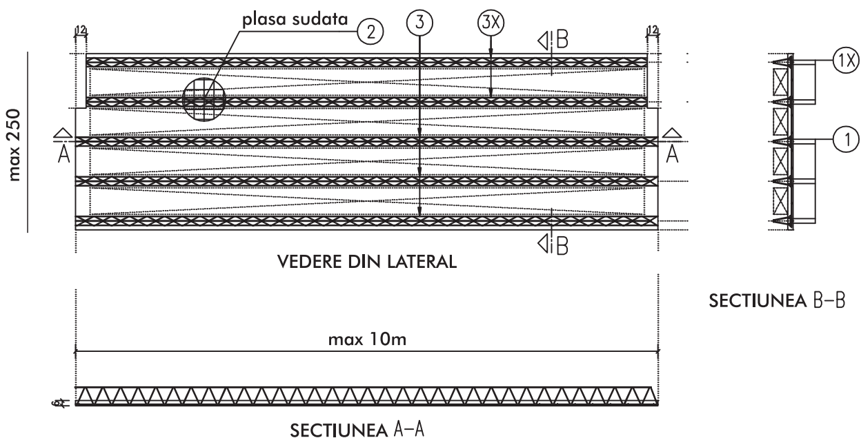
DETALIU PREDALA
