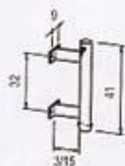
Wandbride 3 oder 15 cm
