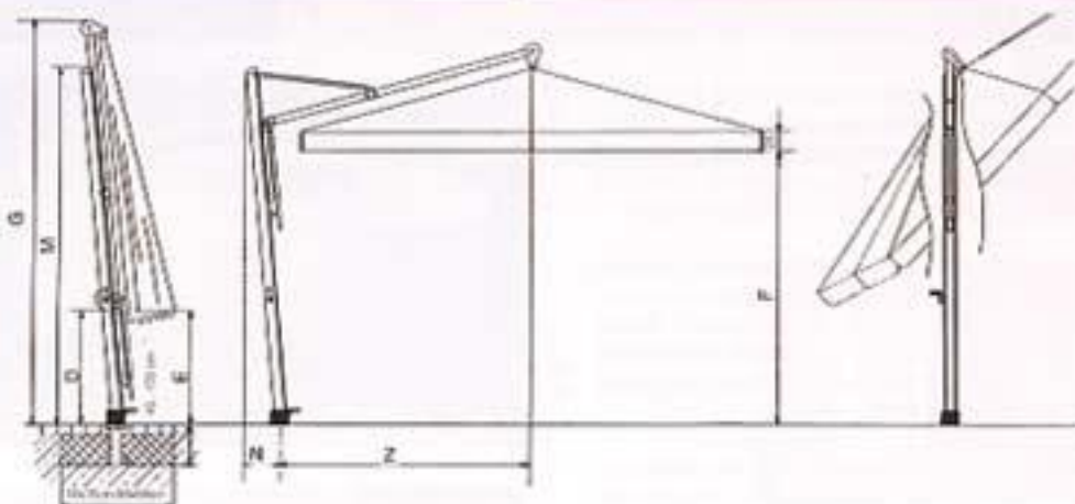
Abbildung: D = Karbonhöhe 95 cm M = Masthöhe 265 cm F = Durchgangshöhe 195 cm N = Auskrüfung 25 cm G = Gesamthöhe 310 cm Z = Länge Trägerr 190 cm
